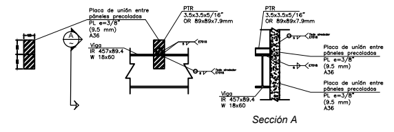
Detalle 1, tipo. Fijación de Fachada Precolada a estructura metálica Nota: este detalle corresponde a cada unión entre pánies de fachada que están a nivel de las Vigas Metálicas W18x60 / IR 457x89.4
